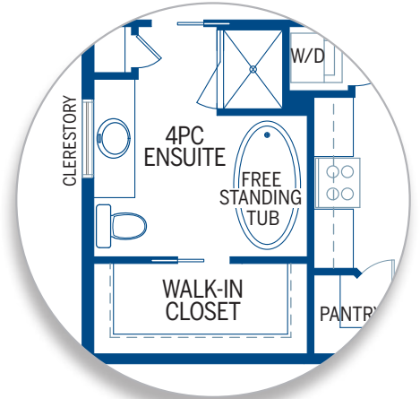
Ensuite Option
